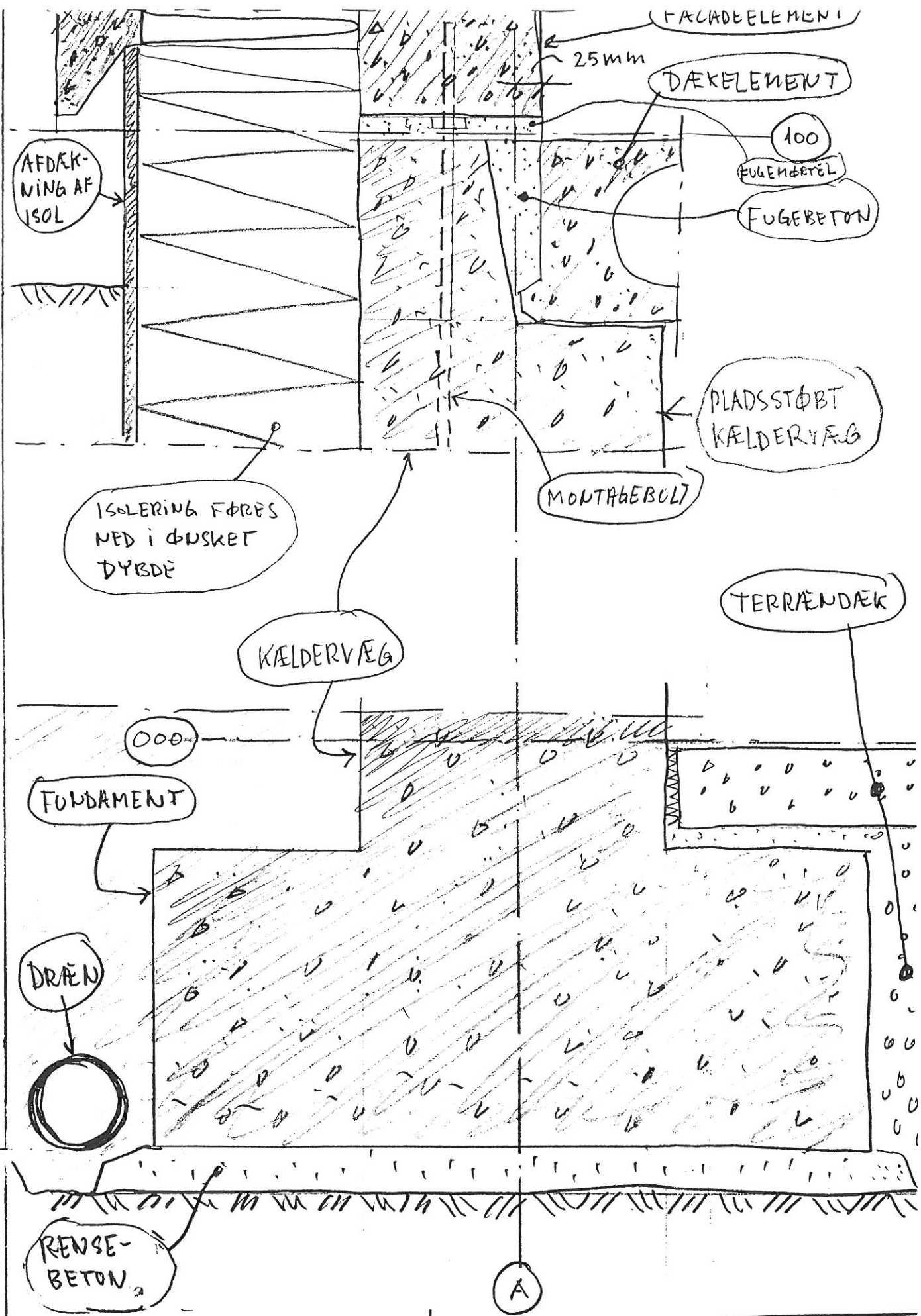
FACADEELEMENTERS TILSLUTNING TIL KÆLDER TEGN. NR B 5 1:5
