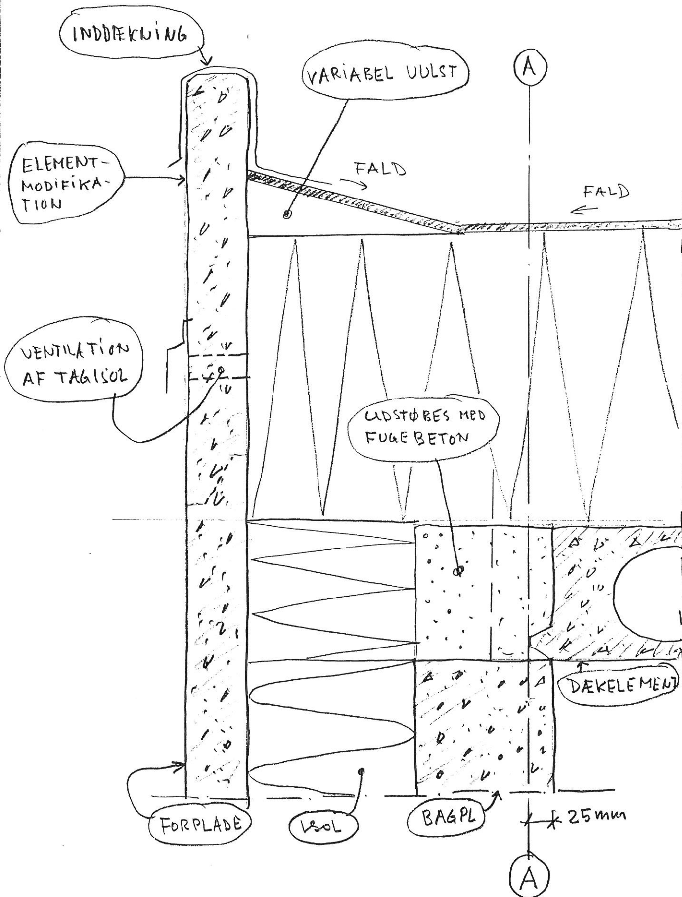
TAGKONSTRUKTION MED FLADT TAG TEGN. NR B 4 1:5
